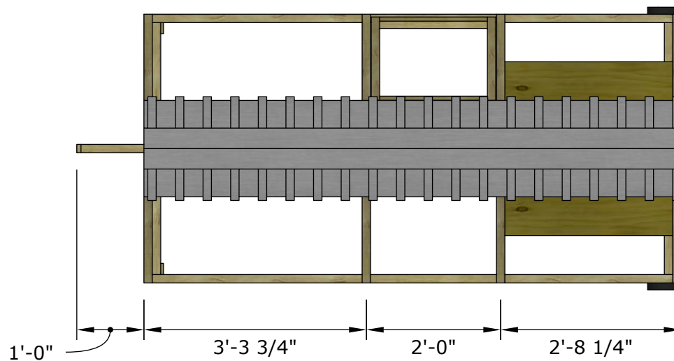
Top Elevation
